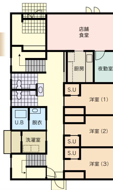
1階 平面図
